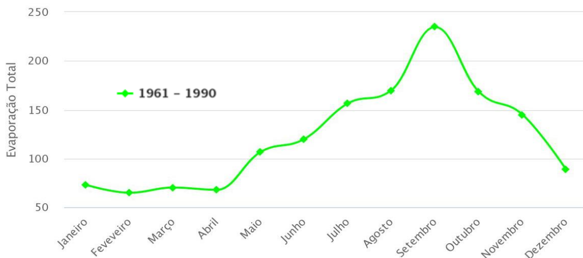
Figura 13. Evaporação, Estação Vale do Gurguéia – Cristino Castro. (Normais Climatológicas INMET).
