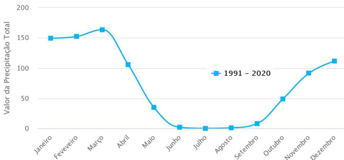
Figura 11. Precipitação Pluviométrica, Estação Vale do Gurguéia-Cristino Castro (Normais Climatológicas INMET).
