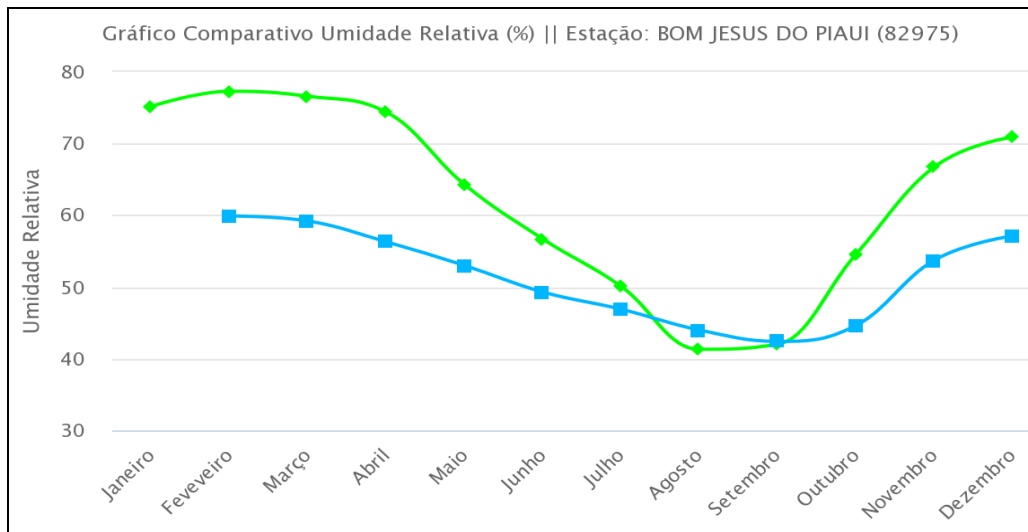
Figura 12. Umidade Relativa, Estação Bom Jesus do Piauí (Normais Climatológicas INMET).
