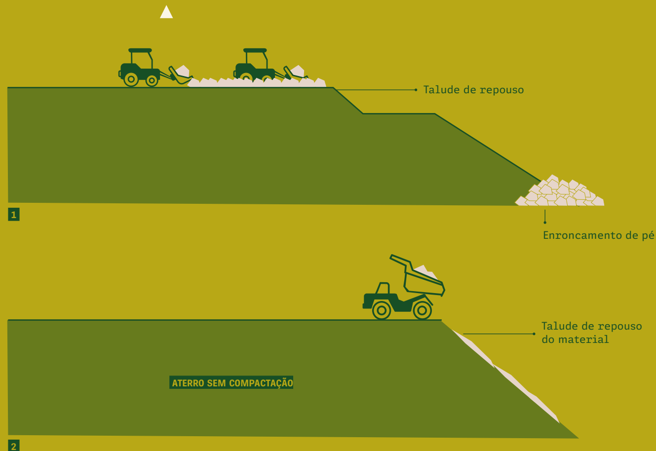
FIGURA 1 Esquema construtivo da pilha de estéril pelo método ascendente. Fonte: Aragão, 2008.
