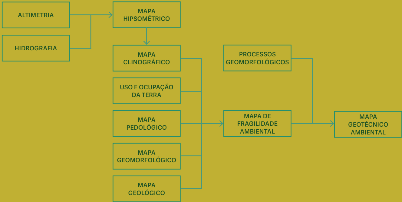
▲ Fluxograma da elaboração do Mapa Geotécnico
