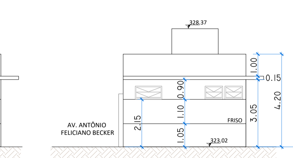
8 FACHADA B ESCALA 1:100
