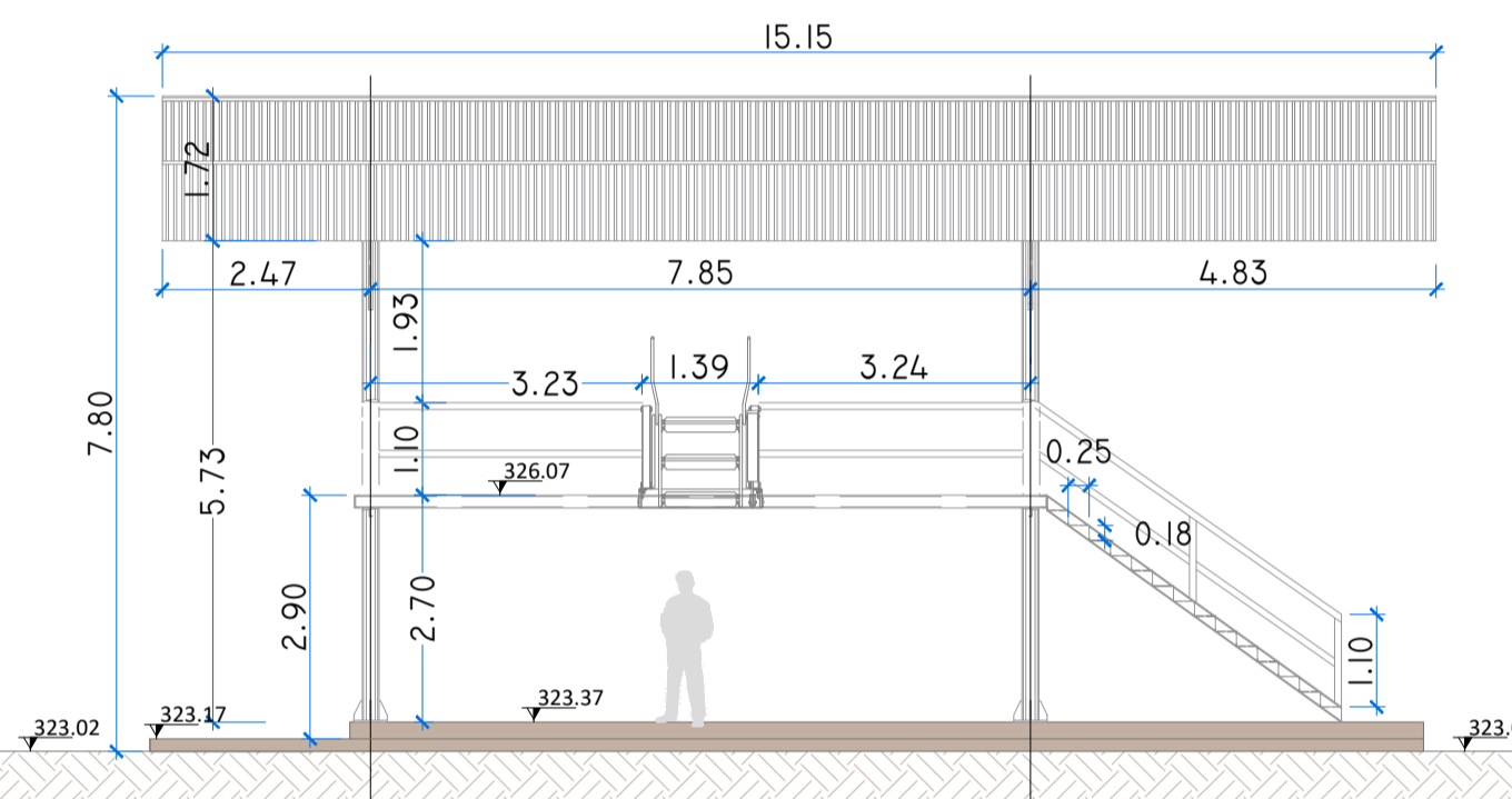
4 CORTE BB ESCALA 1:100
