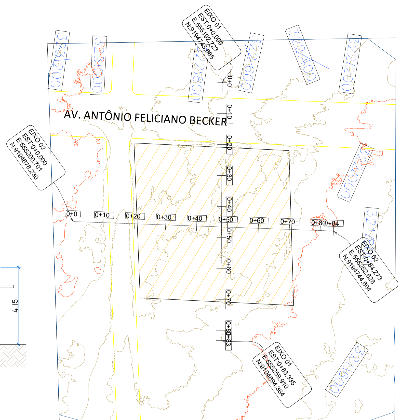
10 PLANTA LEVANTAMENTO TOPOGRÁFICO ESCALA 1:600
