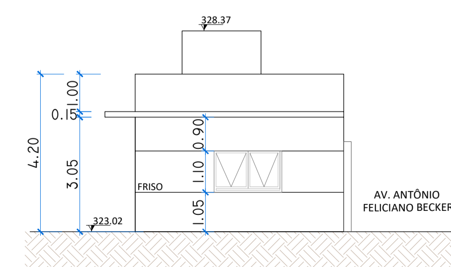
9 FACHADA C ESCALA 1:100
