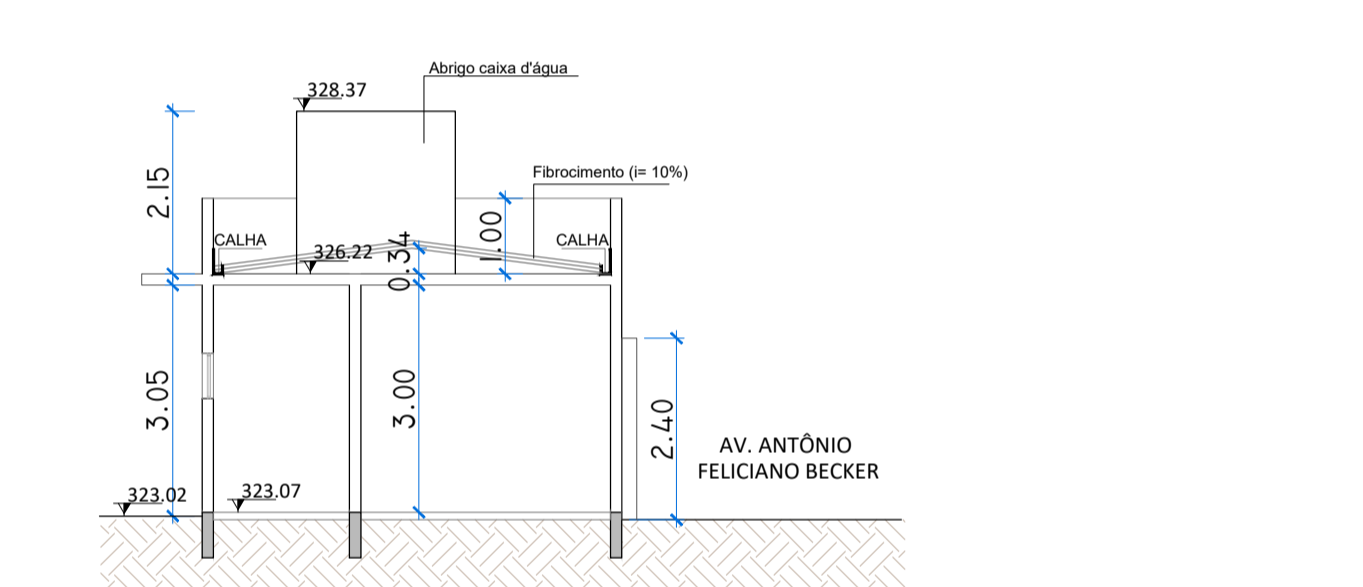
6 CORTE DD ESCALA 1:100
