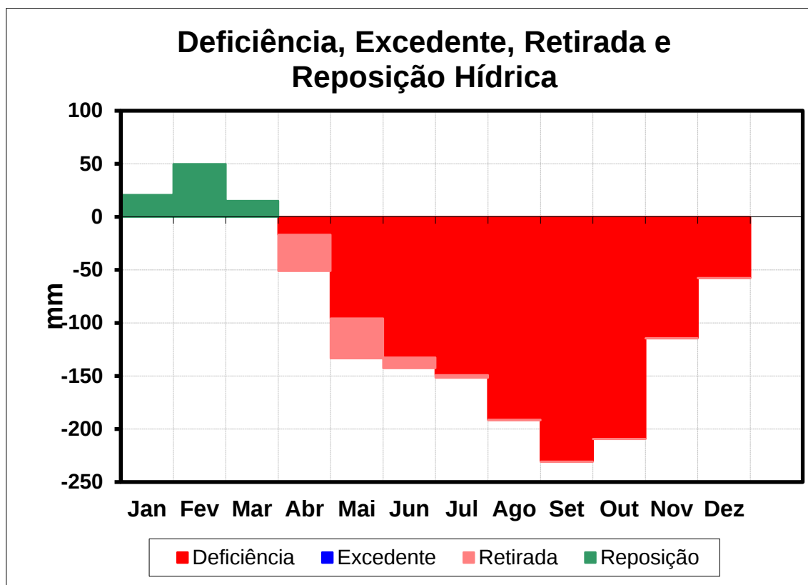
Figura 13. Média da Deficiência hídrica, excedente, retirada e reposição hídrica do município de Flores do Piauí segundo Thornthwaite (1955) de 1991 a 2021.
