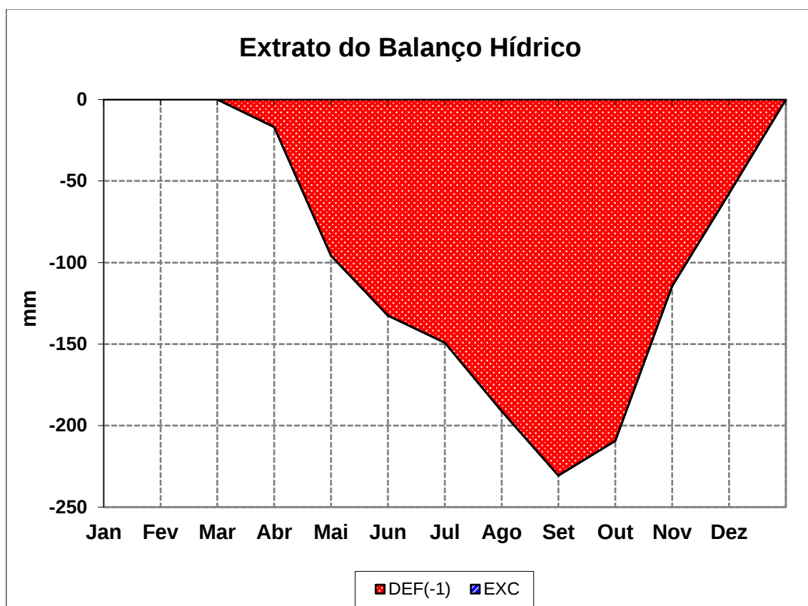
Figura 12. Média anual da Deficiência hídrica do município de Flores do Piauí segundo Thornthwaite (1955) de 1991 a 2021.
