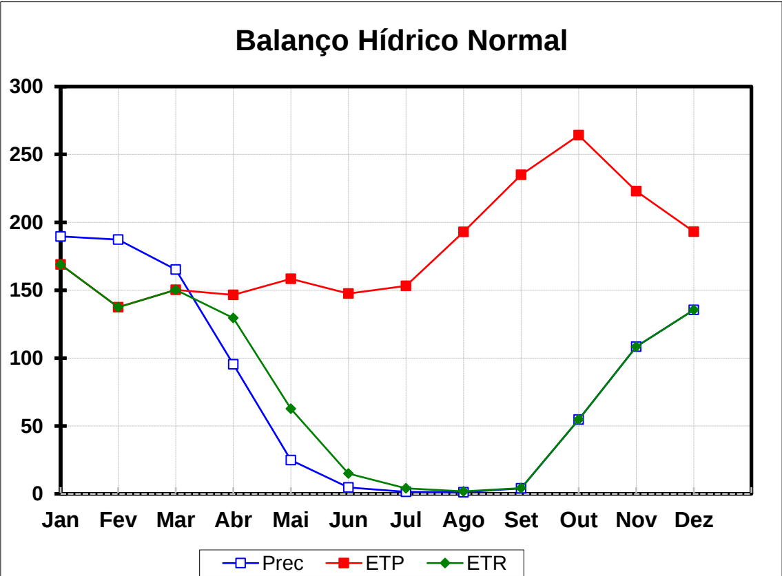
Figura 11. Resultado do Balanço Hídrico de Flores do Piauí, segundo Thornthwaite (1955) de 1991 a 2021.
