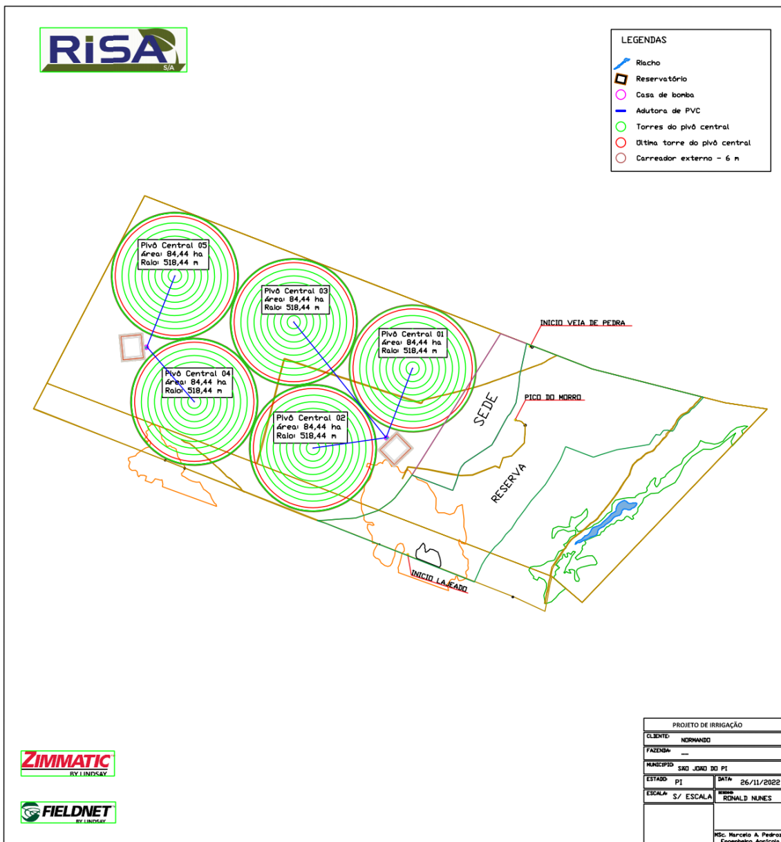
Figura 2. Projeto para irrigação de áreas a serem irrigadas por pivô central.
