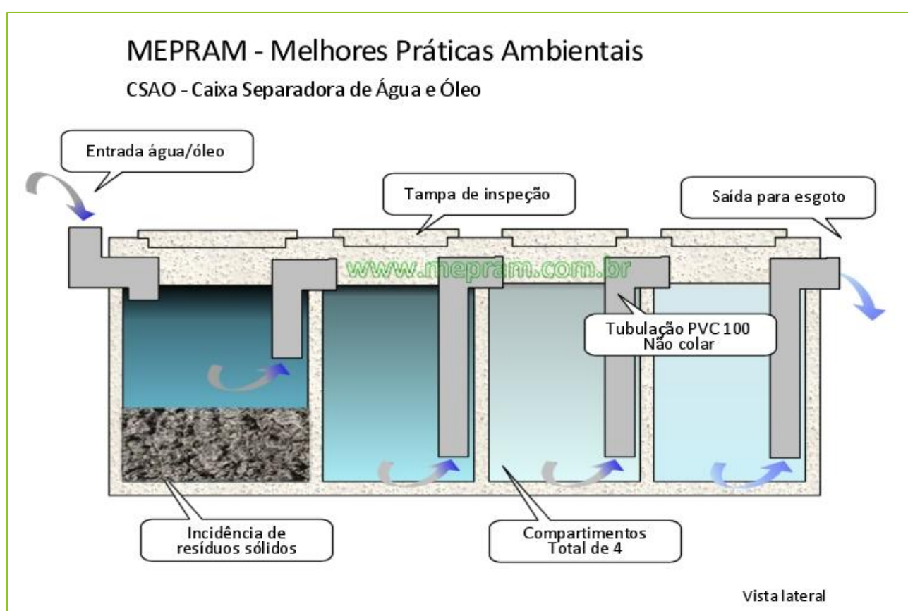
Figura 5. Representação esquemática da Caixa Separadora de Água e Óleo. Fonte: www.mepram.com.br
